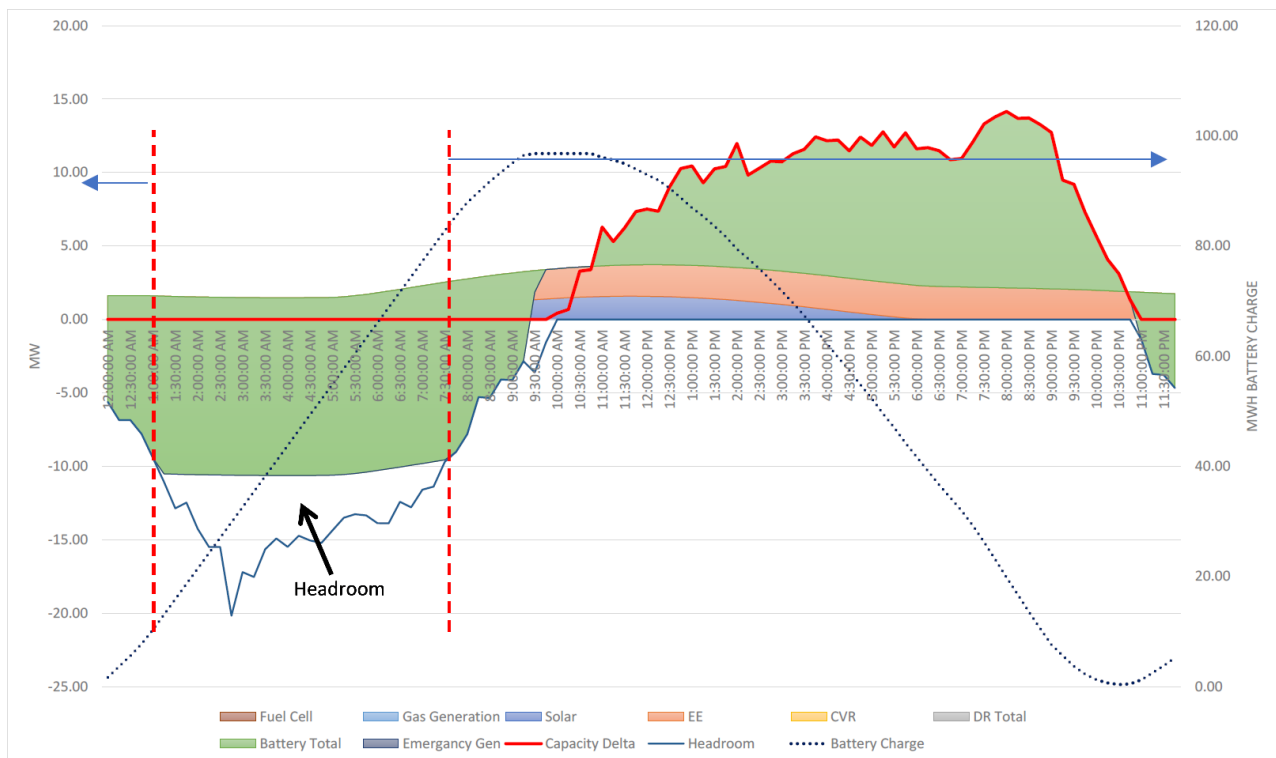
Figura 2: Simulación de despacho en batería en el día punta de 2031 para el área de Chelsea-East Boston.
